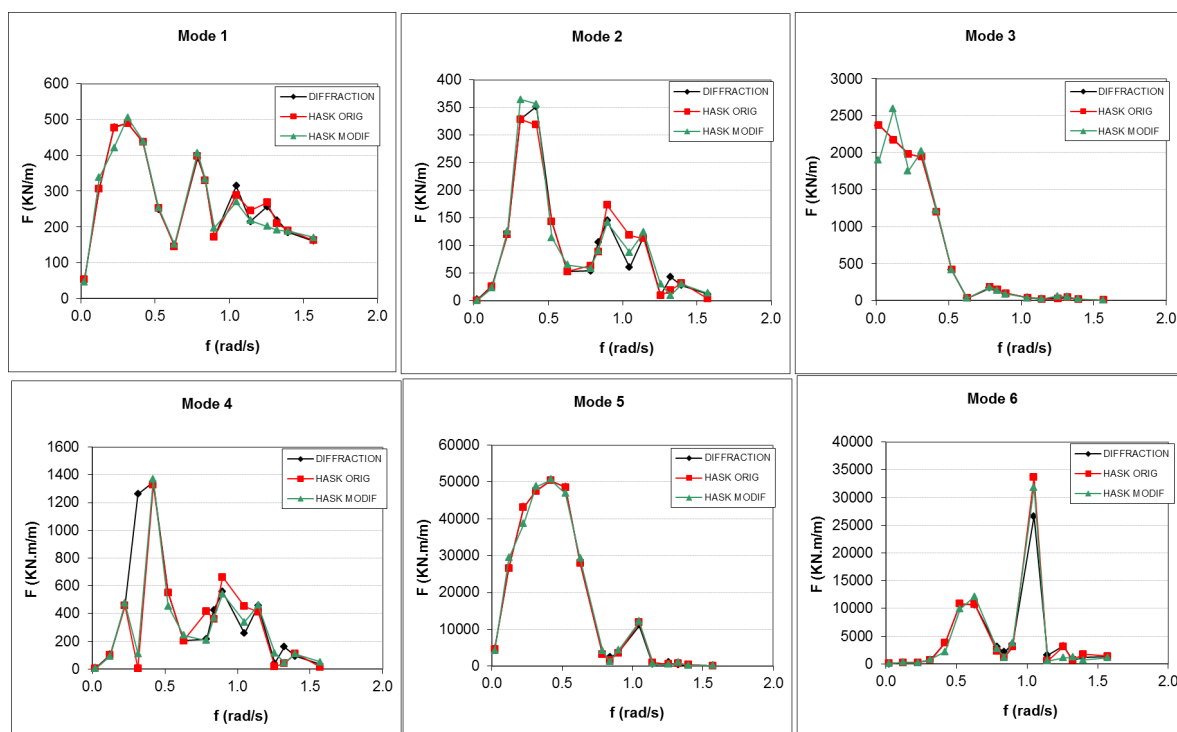
Figura 6. Forças devidas às ondas incidentes ( \theta=90^\circ ) segundo os seis graus de liberdade do navio.
