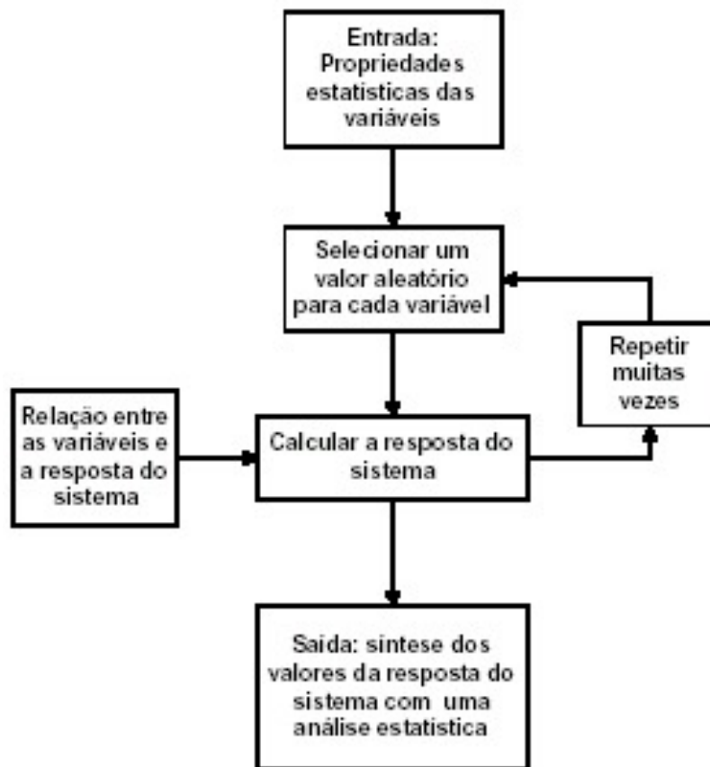
FIGURA 1 – Esquema do funcionamento do método de Monte Carlo [21]
