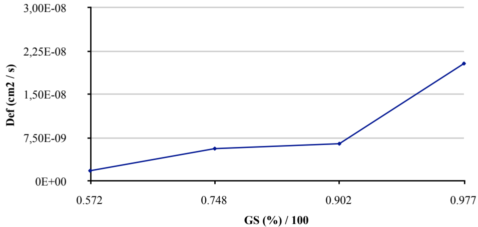
FIGURA 2 - Coeficiente de difusão efetivo em função do GS e a relação entre o maior coeficiente de difusão e os demais valores
