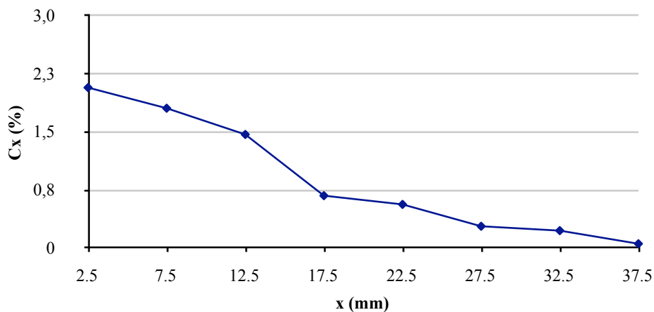
FIGURA 3 – Perfil de teor de íons cloreto
