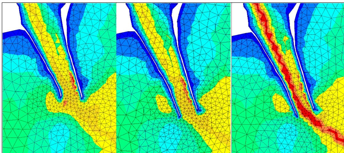
Figura 5 – Cenários sob investigação: A) configuração atual; B) extensão dos molhes; C) extensão e aprofundamento do canal para 20m.
